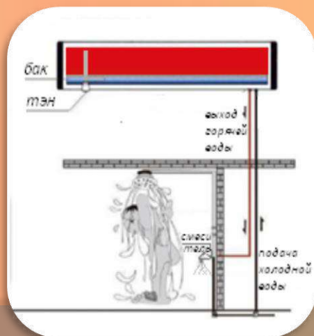
Схема солнечного водонагревателя без давления (термосифонная система)
